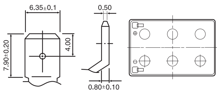
Faston tab : 250
