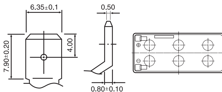
Faston tab : 250
