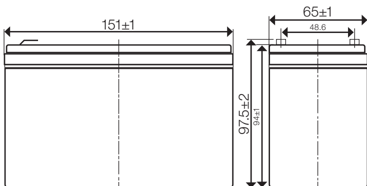
Faston tab : 250
